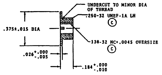
-3, -6 FLANGE
